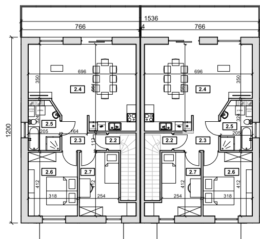
Piętro
